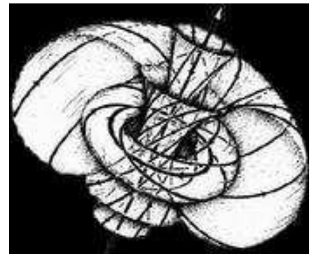
Wirbelmodell eines Photons nach Roger Penrose.
