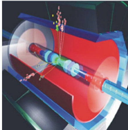
Partikel-Dektoren am DESY, mit denen die Eigenschaften der Elementarteilchen gemessen werden.
